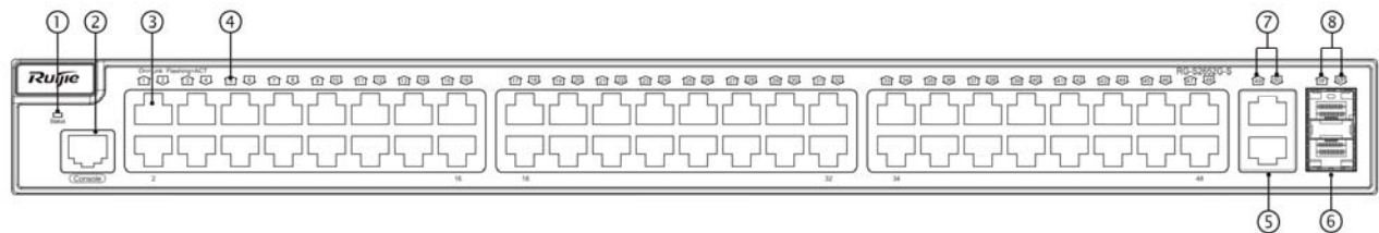
图 1-5 RG-S2652G-S 前面板示意图
