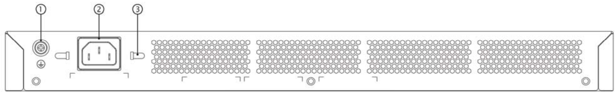
图 1-3 RG-S2628G-S 后面板示意图
